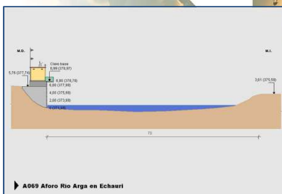
Ilustración 5. Esquema y vista de la estación de aforo de la Confederación Hidrográfica del Ebro (CHE) en el río Arga en Etxauri (A069).
