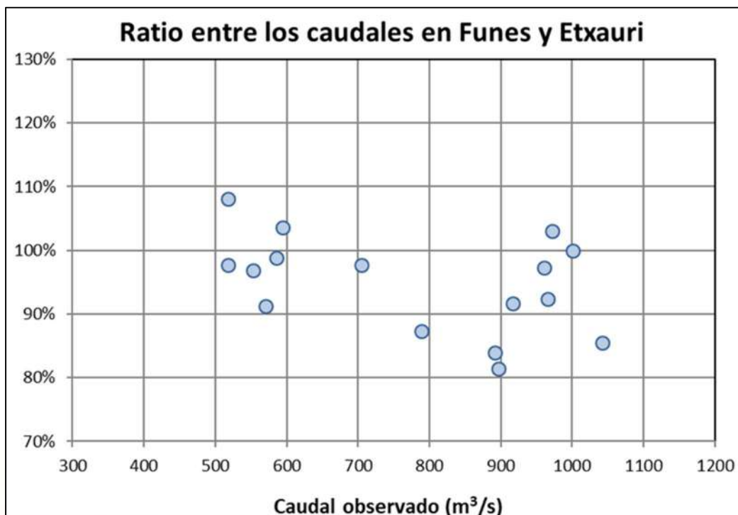
Ilustración 37. Ratio entre el caudal pico observado en la E.A. de Funes y el que circuló para cada evento por la E.A. de Etxauri. Se han añadido los datos de los eventos de diciembre 2021 y enero 2022.
