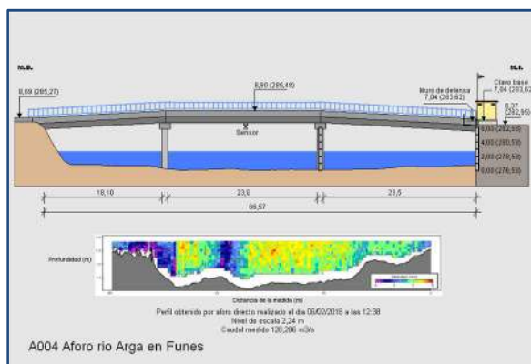
Ilustración 6. Esquema y vista de la estación de aforo de la CHE en el río Arga en Funes (A004).
