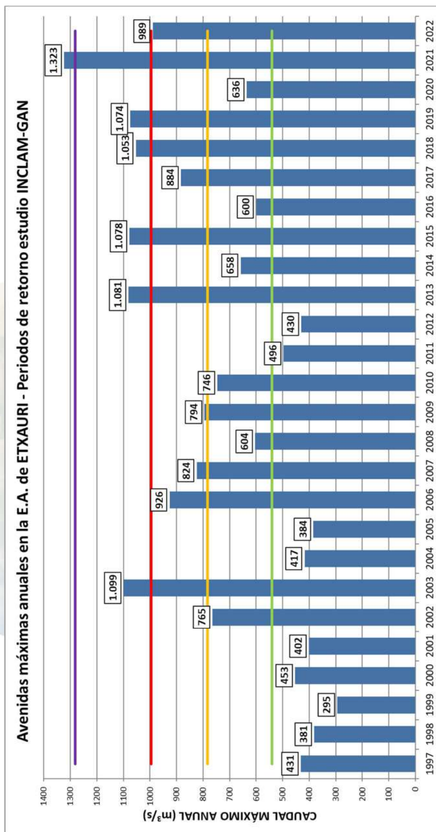
Ilustración 13. Caudales máximos instantáneos observados en cada uno de los últimos 26 años en la estación de aforo del Arga en Etxauri. Periodo 1997-2022. Las líneas horizontales marcan los caudales asociados a los periodos de retorno de 2,3 (540 m³/s), 5 (782 m³/s), 10 (996 m³/s) y 25 años (1282 m³/s).
