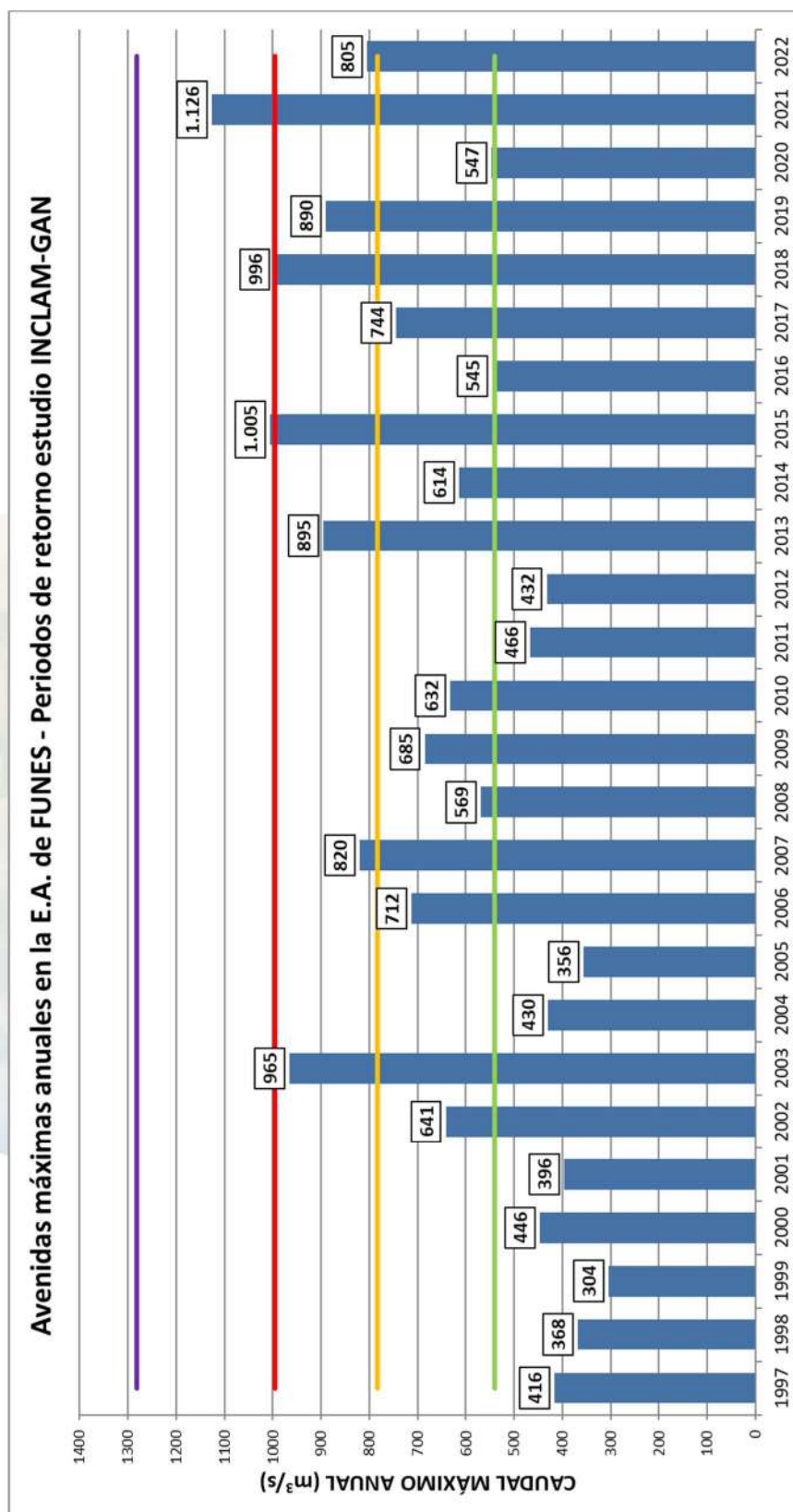
Ilustración 14. Caudales máximos instantáneos observados en cada uno de los últimos 26 años en la estación de aforo del Arga en Funes. Periodo 1997-2022. Las líneas horizontales marcan los caudales asociados a los periodos de retorno de 2,3 (540 m³/s), 5 (782 m³/s), 10 (996 m³/s) y 25 años (1282 m³/s).
