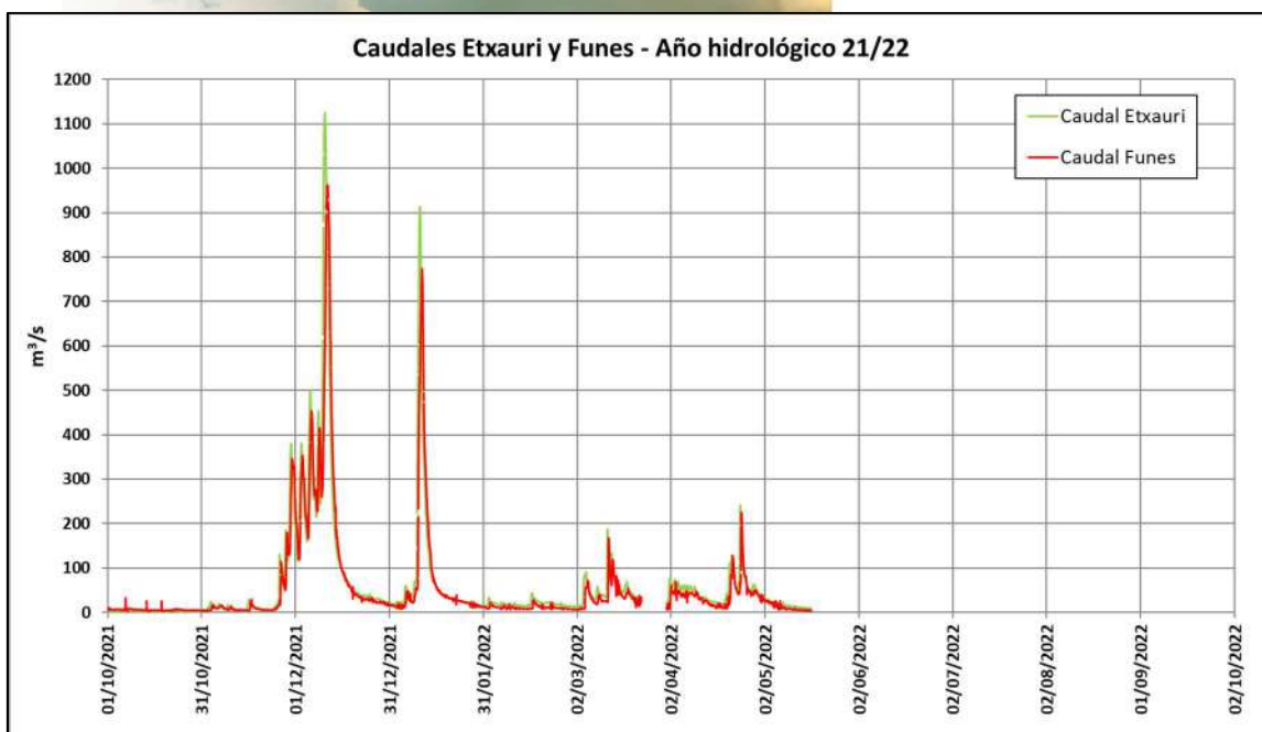
Ilustración 21. Datos históricos observados en las estaciones de aforo de Etxauri y Funes. Año hidrológico 21-22. Grafico añadido en la segunda versión del plan.
