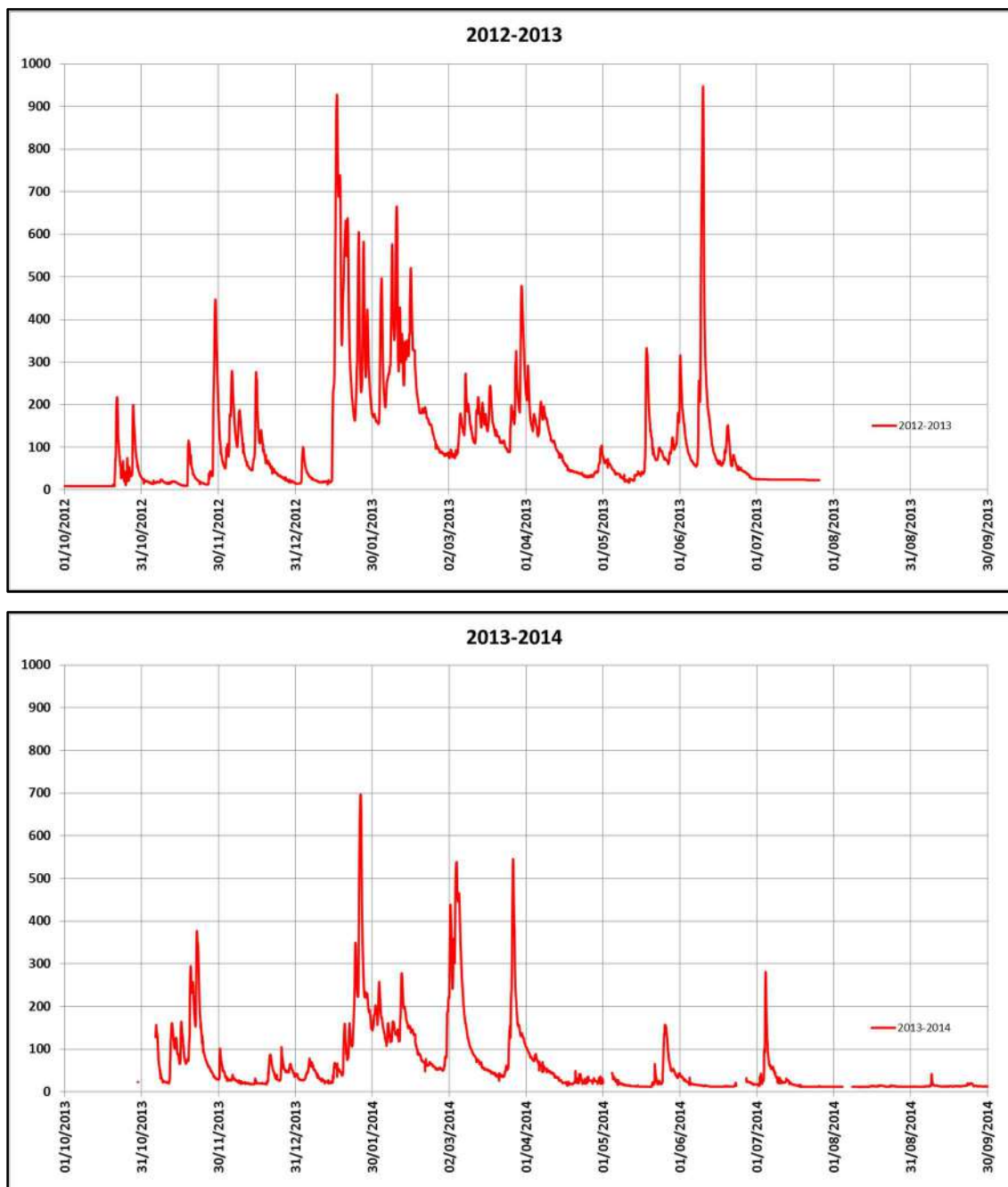
Ilustración 15. Datos históricos observados en la estación de aforo de Funes. Año hidrológico 12-13. Año hidrológico 13-14.
