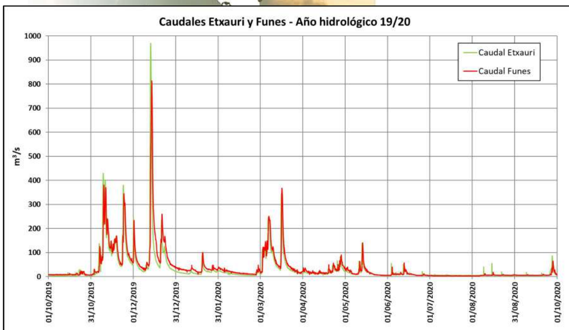
Ilustración 19. Datos históricos observados en las estaciones de aforo de Etxauri y Funes. Año hidrológico 19-20. Grafico añadido en la segunda versión del plan.
