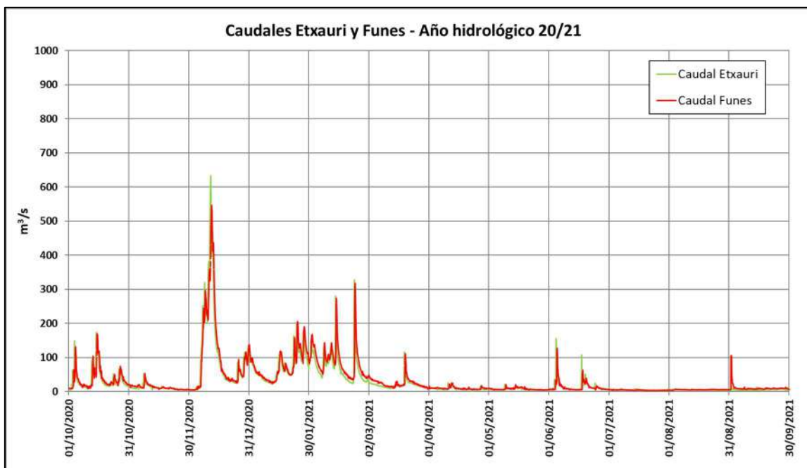
Ilustración 20. Datos históricos observados en las estaciones de aforo de Etxauri y Funes. Año hidrológico 20-21. Grafico añadido en la segunda versión del plan.
