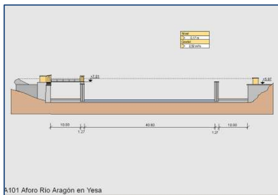
Ilustración 8. Estación de aforo del río Aragón en Yesa Pie de Presa, propiedad de la CHE (Código A101). Foto y esquema obtenidos de: www.saihebro.com
