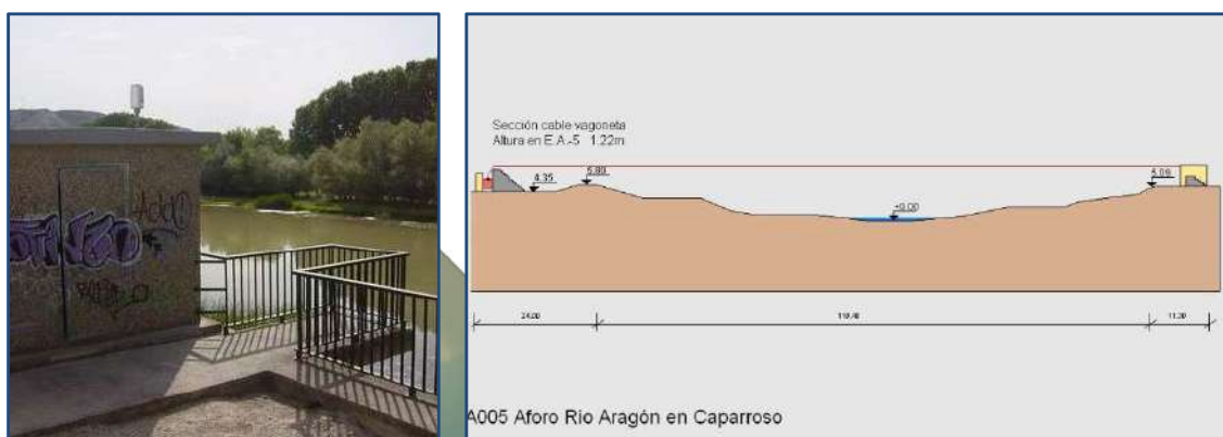
Ilustración 11. Estación de aforo del río Aragón en Caparroso, propiedad de la CHE (Código A005). Foto y esquema obtenidos de: www.saihebro.com
