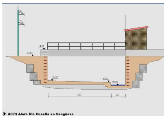
Ilustración 9. Estación de aforo del río Onsella en Sangüesa, propiedad de la CHE (Código A073). Foto y esquema obtenidos de: www.saihebro.com
