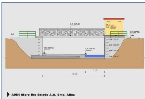
Ilustración 4. Esquema y vista de la estación de aforo de la CHE en el río Salado, en Alloz, aguas abajo del embalse (A084).
