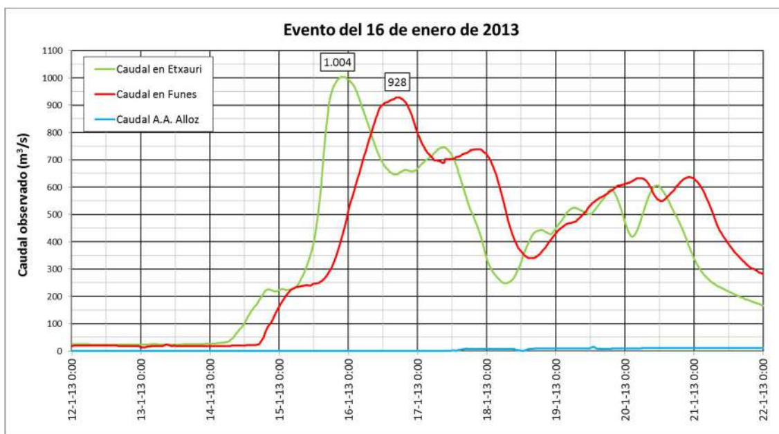
Ilustración 39. Caudales observados en la cuenca baja del río Arga durante el evento ocurrido los días 15 y 16 de enero de 2013.
