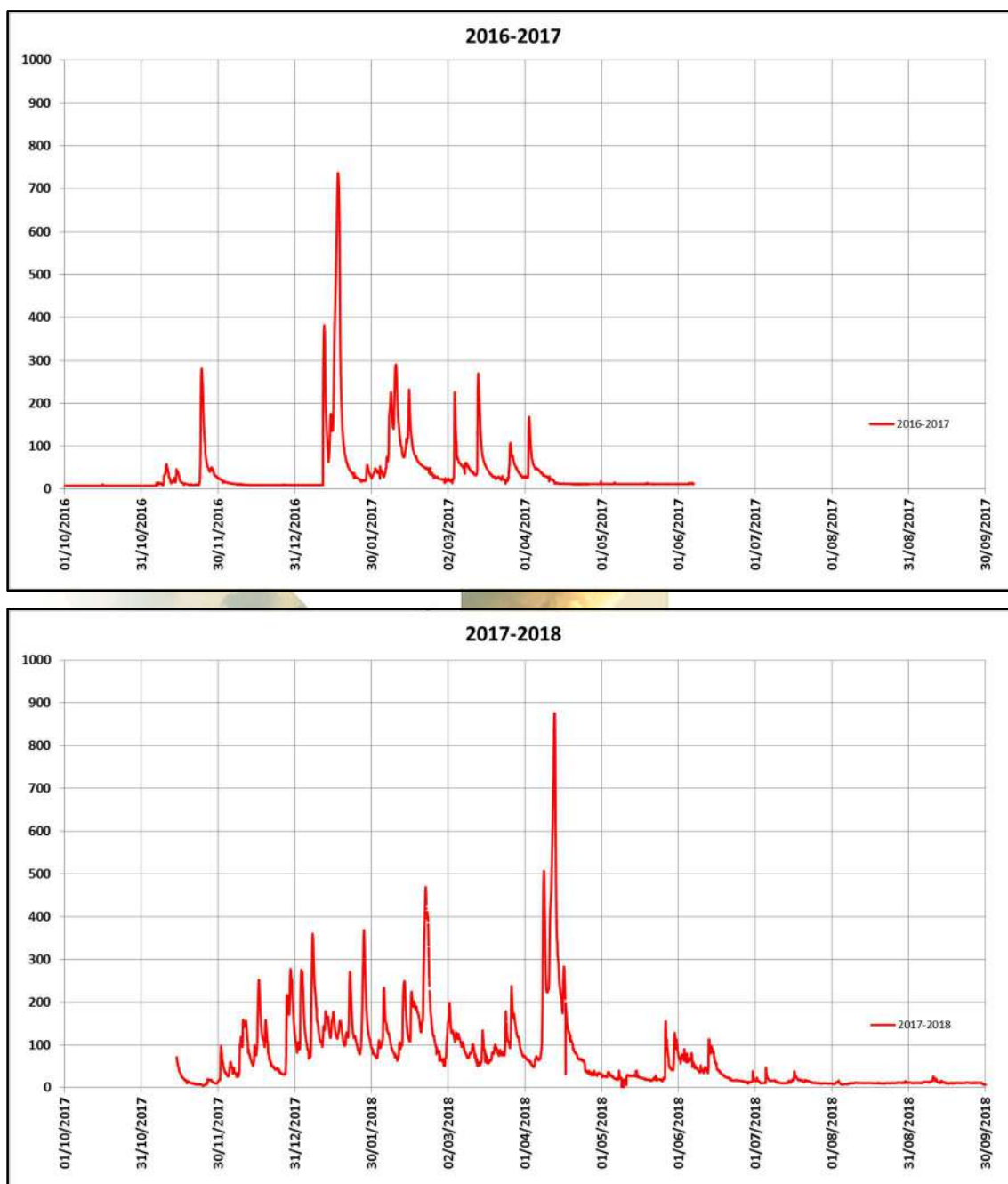
Ilustración 17. Datos históricos observados en la estación de aforo de Funes. Año hidrológico 16-17. Año hidrológico 17-18.
