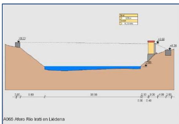
Ilustración 7. Estación de aforo del río Irati en Liédena, propiedad de la CHE (Código A065). Foto y esquema obtenidos de: www.saihebro.com
