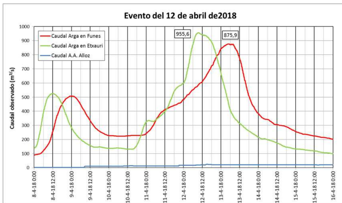
Ilustración 40. Caudales observados en la cuenca baja del río Arga durante el evento ocurrido los días 24 y 12 de abril de 2018.
