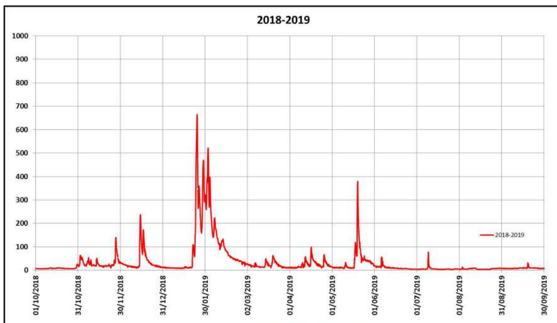
Ilustración 18. Datos históricos observados en la estación de aforo de Funes. Año hidrológico 18-19.
